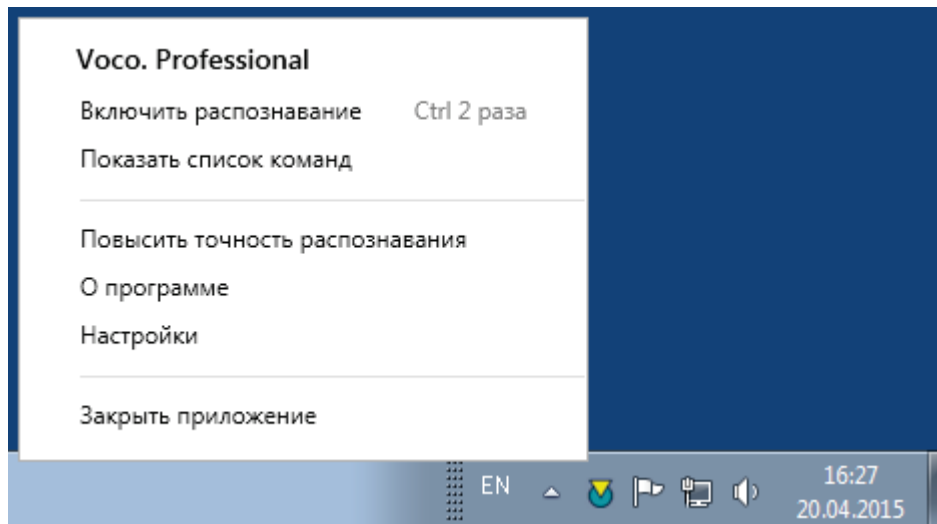
Рисунок 13 – Вызов меню
