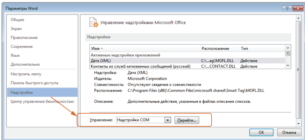
Рисунок 69 – Надстройки Word
