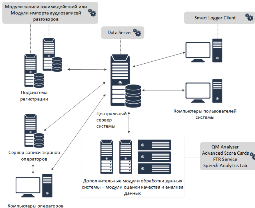
Рисунок 1 – Типовая схема развёртывания системы
